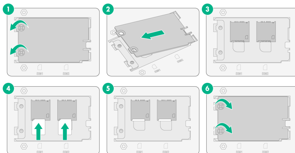
图1-11 安装 5G SIM 卡
